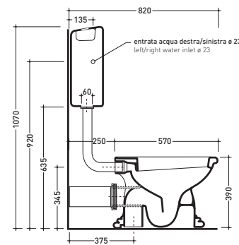
sezione longitudinale / section
