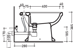
sezione longitudinale / section
